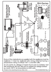
Wiring Label
